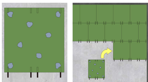
Bodové nanášení lepidla na zadní stěnu desky, pokládka desky
